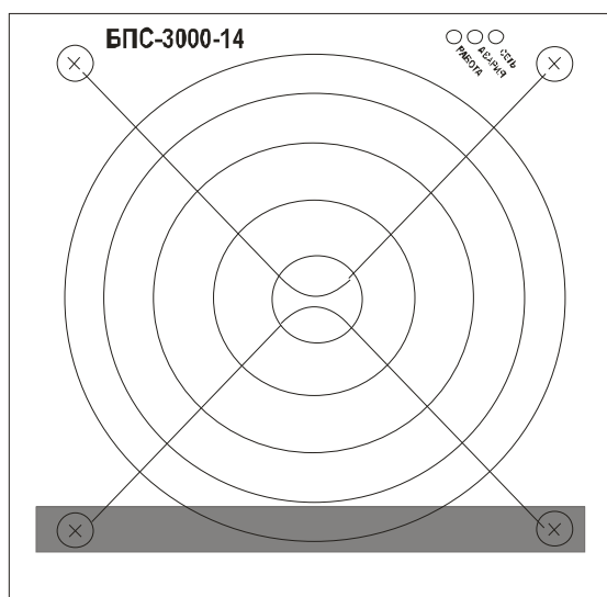
Рис.2. Вид БПС спереди.
